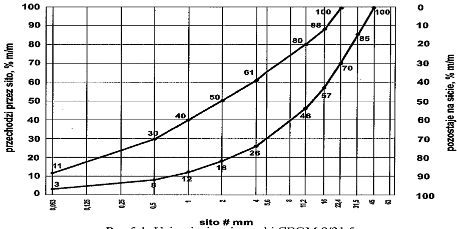
Rys. 5.1. Uziarnienie mieszanki CBGM 0/31,5
