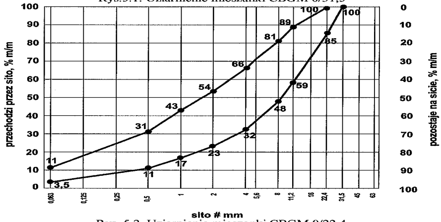
Rys. 5.2. Uziarnienie mieszanki CBGM 0/22,4
